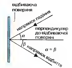
Відбивач
